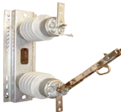
Cuchilla Monopolar Loadbuster Disconnects estilo Branch Feeder (para derivaciones)
